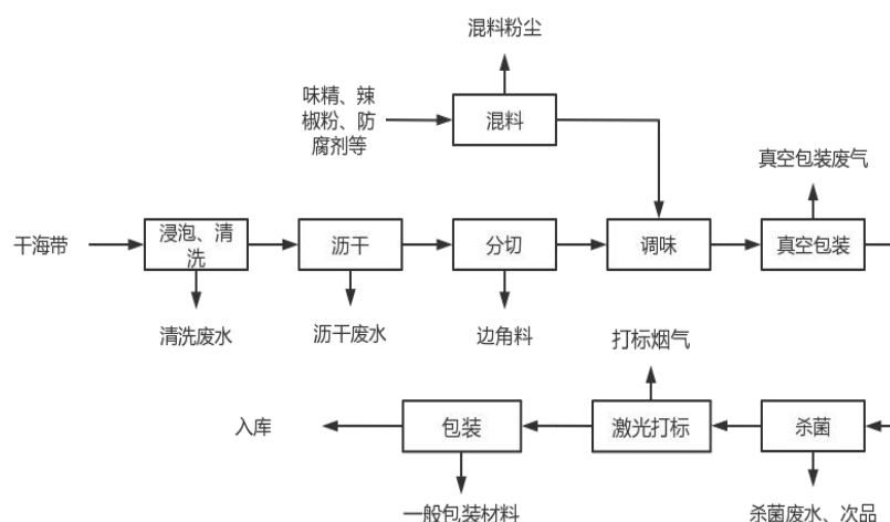
图 2-3 本项目盐渍水产品生产工艺流程图（各工序均有噪声产生）
