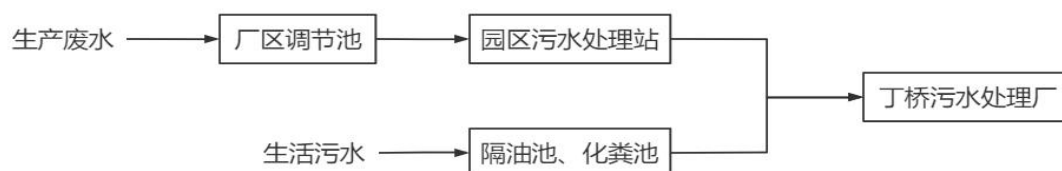
图 4-1 废水纳管图
