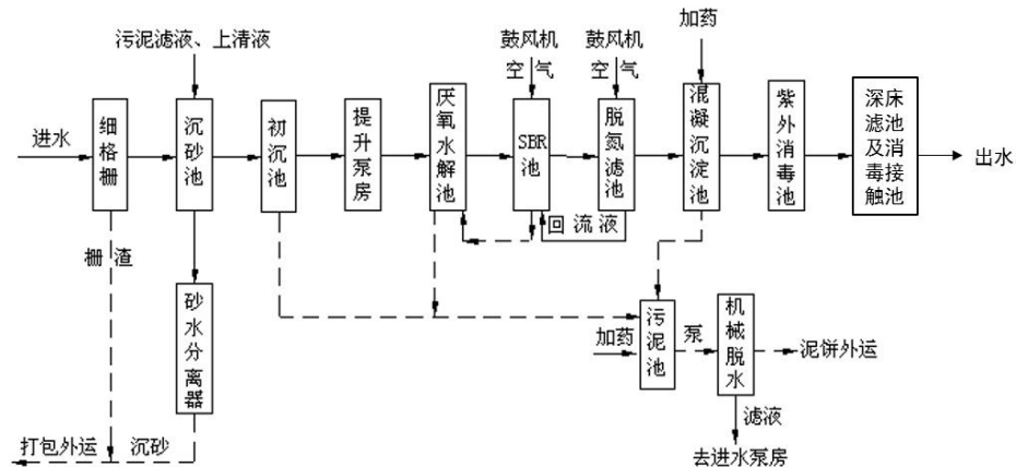
图 4-3 污水处理厂一期、二期废水处理工艺
