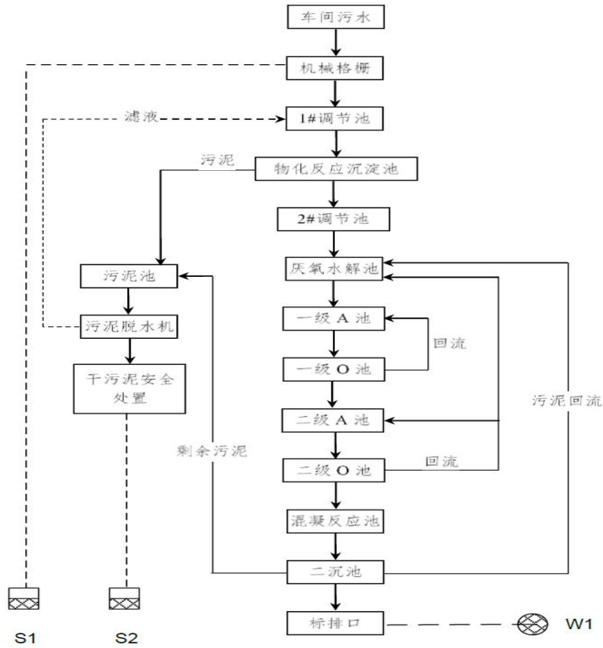
图 4-2 污水处理工艺图
