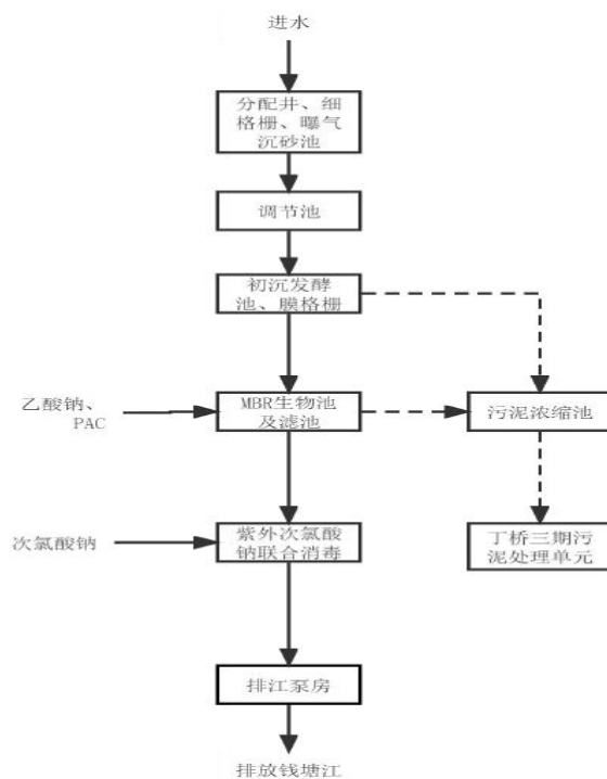
图 4-5 污水处理厂四期现状废水处理工艺
