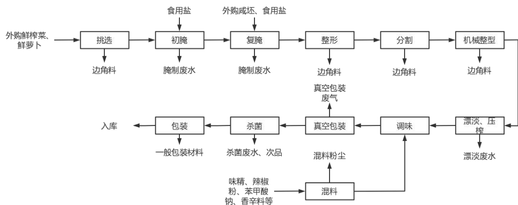
图 2-2 本项目酱腌菜生产工艺流程图（各工序均有噪声产生）
