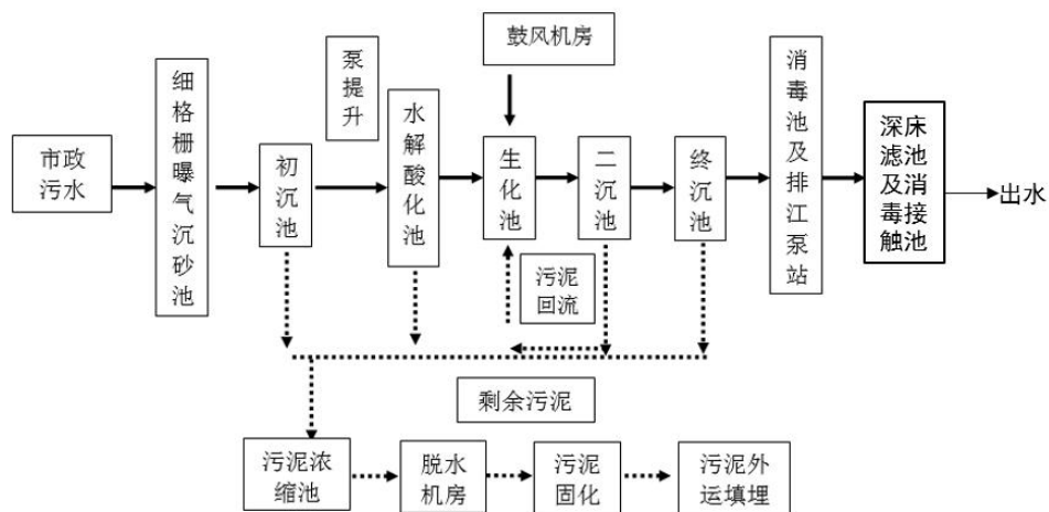
图 4-4 污水处理厂三期废水处理工艺
